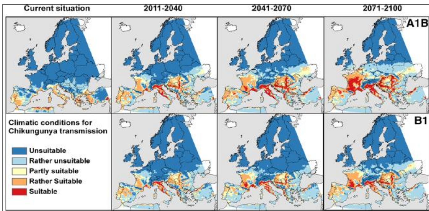
Εικόνα B20: Χάρτες επικινδυνότητας για τη μετάδοση του ιού Chikungunya στην Ευρώπη στο παρόν αλλά και με βάση τα κλιματικά σενάρια SRES-A1B και SRES-B1 (Πηγή: Fischer et al, 2013)
