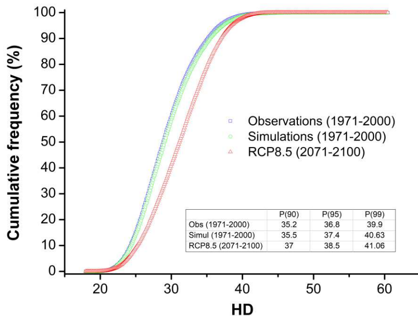
Εικόνα Γ10: Αθροιστική συχνότητα κατανομής (CDF) του HD (Humidex) για την περίοδο αναφοράς (1971–2000) με βάση τα δεδομένα επίγειων παρατηρήσεων και προσομοιώσεων καθώς και προβολή του HD στο απώτερο μέλλον (2071–2100) βάσει προσομοιώσεων υπό το μελλοντικό σενάριο εκπομπών RCP8.5 στην Αθήνα.
