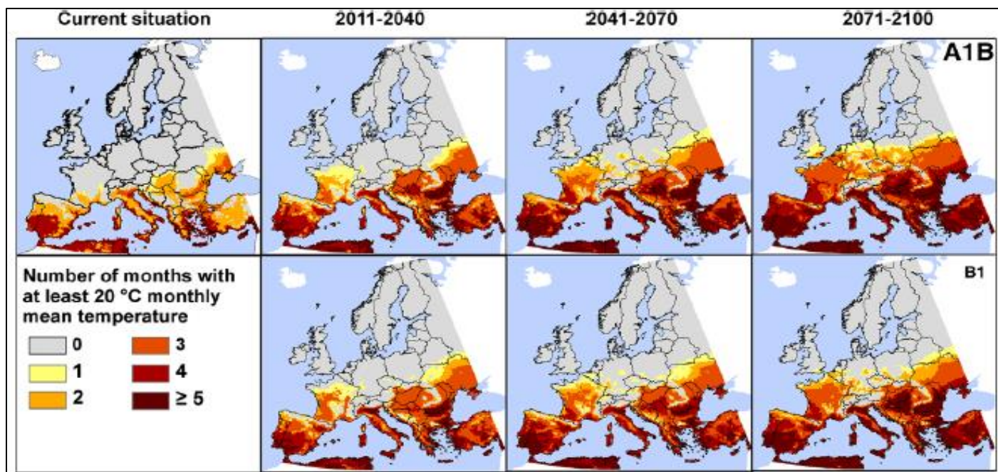
Εικόνα B21: Χάρτες της Ευρώπης που παρουσιάζουν το κατά τόπους πλήθος των μηνών στους οποίους καλύπτεται το κριτήριο για μέση θερμοκρασία άνω των 20°C, το οποίο είναι αναγκαίο για τη δράση του ιού Chikungunya, στο παρόν αλλά και με βάση τα κλιματικά σενάρια SRES-A1B και SRES-B1 (Πηγή: Fischer et al, 2013)
