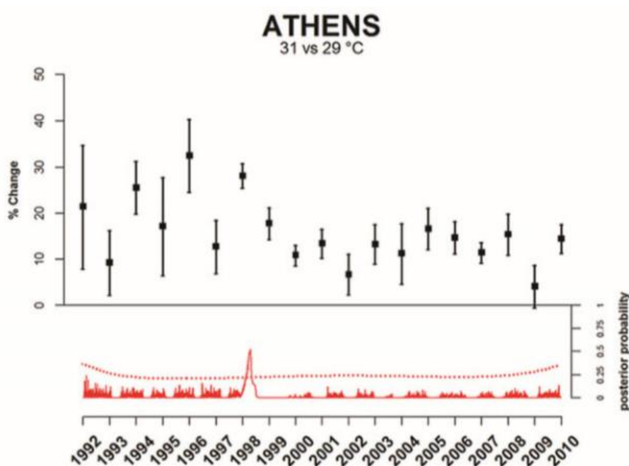
Εικόνα A9: Επίδραση της θερμοκρασίας περιβάλλοντος στη θνησιμότητα στην Αθήνα ανά έτος για την περίοδο 1992-2010. Άνω γράφημα: Επιδράσεις που εκφράζονται ως ποσοστιαία μεταβολή της θνησιμότητας για αύξηση κατά 2 °C της μέσης θερμοκρασίας πέραν του ορίου (29 °C). Κάτω γράφημα: Ύστερη πιθανότητα ενός σημείου αλλαγής κάθε εκτιμώμενης παρατήρησης από την ανάλυση Bayesian Change Point. Η κόκκινη διακεκομμένη γραμμή αντιπροσωπεύει τη στατιστική σημαντικότητα (Πηγή: Scortichini et al., 2018).
