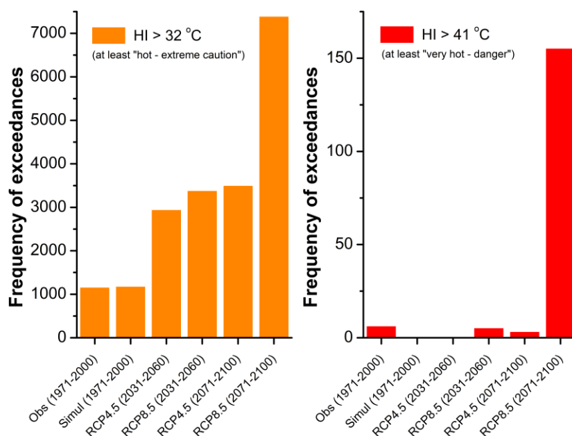
Εικόνα Γ22: Συχνότητα υπερβάσεων (απόλυτος αριθμός 3-ωρων) όταν HI > 32\text{ }^{\circ}\text{C} (τουλάχιστον «πολύ ζεστό – εξαιρετική προσοχή») και HI > 41\text{ }^{\circ}\text{C} (τουλάχιστον «πάρα πολύ ζεστό – κίνδυνος») για την περίοδο αναφοράς (1971–2000) με βάση τα δεδομένα επίγειων παρατηρήσεων και προσομοιώσεων καθώς και προβολή του HI στο εγγύς (2031–2060) και απώτερο (2071–2100) μέλλον βάσει προσομοιώσεων υπό τα μελλοντικά σενάρια εκπομπών RCP4.5 και RCP8.5 στη Θεσσαλονίκη.
