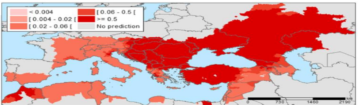
Εικόνα B17: Χάρτες εκτιμώμενης πιθανότητας για τη ύπαρξη αυτόχθονων κρουσμάτων του ιού του Δυτικού Νείλου σε περιοχές της Ευρώπης και γειτονικών χωρών α) για το έτος 2025 β) για το έτος 2050 (Πηγή: Semenza et al, 2016)
