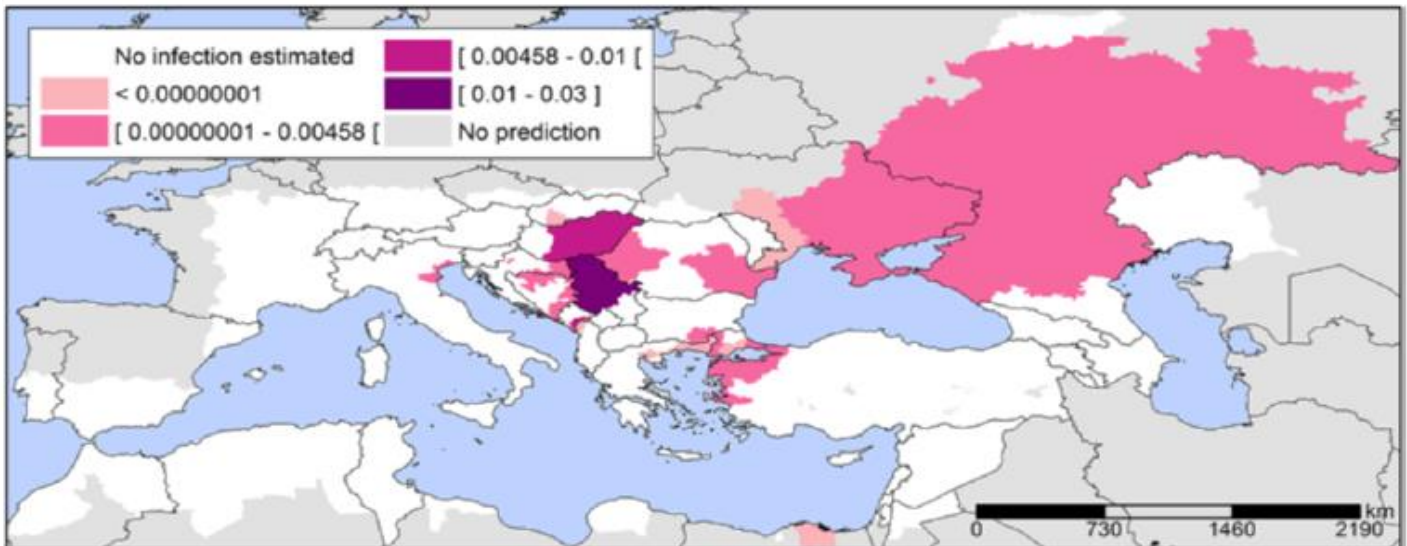
Εικόνα Β18: Χάρτες εκτιμώμενων αυτόχθονων κρουσμάτων του ιού του Δυτικού Νείλου στον πληθυσμό των αιμοδότην (ανά 100000) σε περιοχές της Ευρώπης και γειτονικών χωρών α) για το έτος 2014 β) για το έτος 2025 (Πηγή: Semenza et al, 2016)
