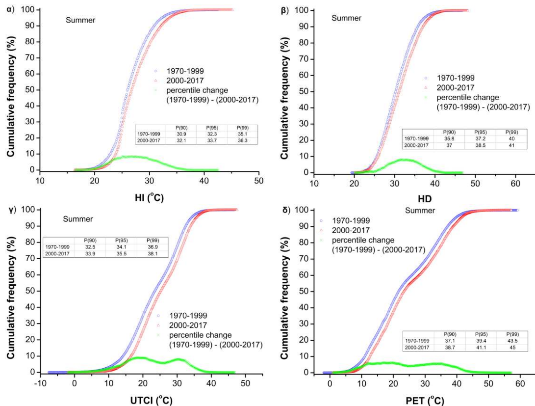
Εικόνα Γ15: Αθροιστική συχνότητα κατανομής (CDF) των δεικτών α) HI, β) HD, γ) UTCI και δ) PET κατά τις δύο υποπεριόδους 1970–1999 και 2000–2017 το καλοκαίρι στη Θεσσαλονίκη. Η εκατοστημιαία μεταβολή (percentile change) μεταξύ των υπό εξέταση υποπεριοδών απεικονίζεται επίσης.
