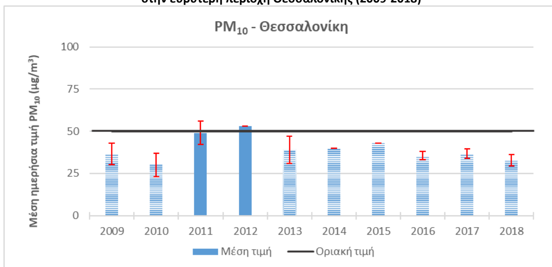
Γράφημα 46: Μέση ημερήσια συγκέντρωση PM_{10} των σταθμών υποβάθρου στην ευρύτερη περιοχή Θεσσαλονίκης (2009-2018)
