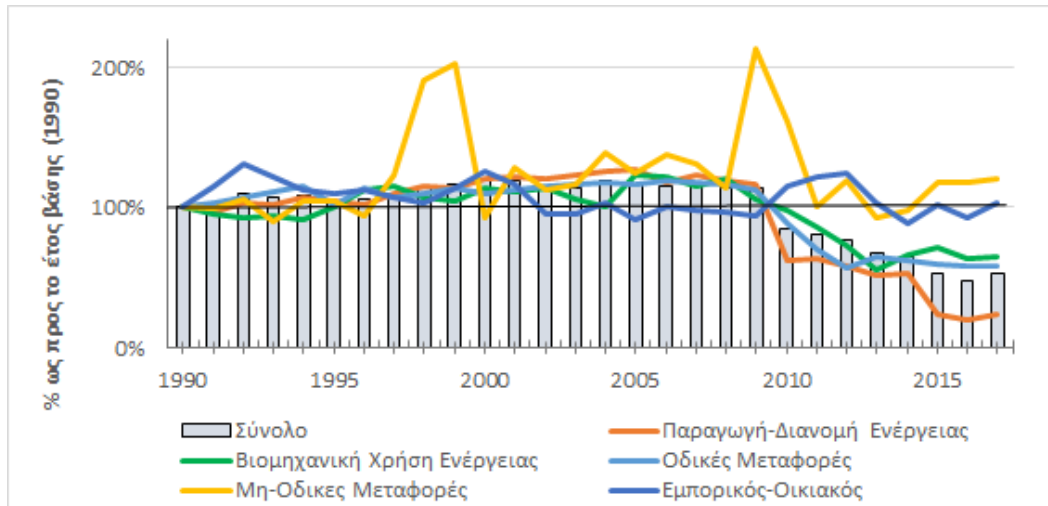
Γράφημα 18: Διαχρονική μεταβολή εκπομπών πρωτογενών PM 10 που σχετίζονται με την ενέργεια, ανά τομέα
