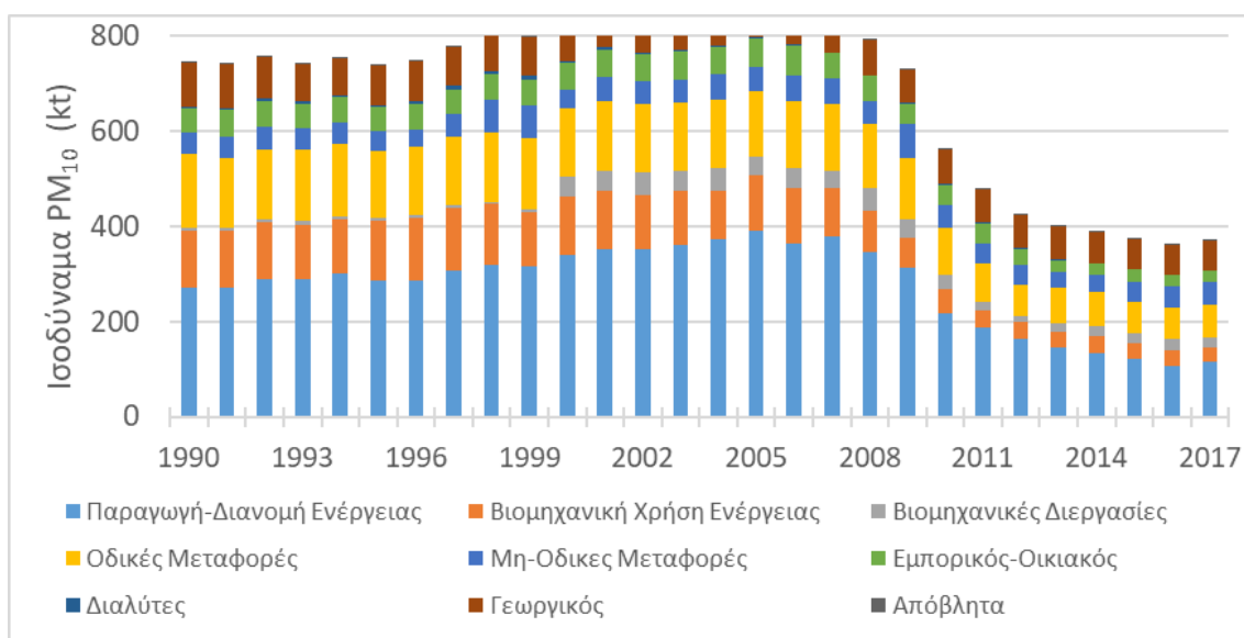
Γράφημα 14: Διαχρονική εξέλιξη των εκπομπών πρωτογενών σωματιδίων PM 10 στην Ελλάδα
