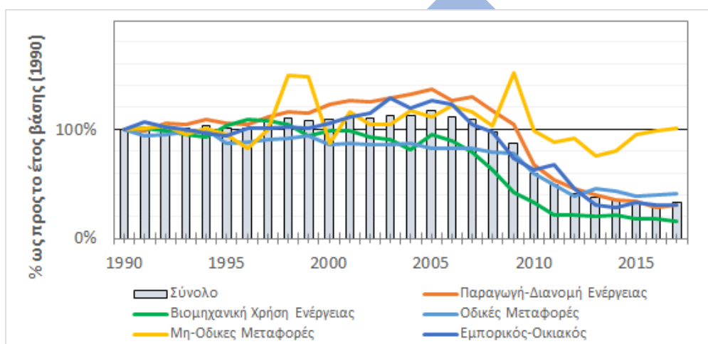
Γράφημα 23: Διαχρονική μεταβολή εκπομπών ουσιών οξίνισης που σχετίζονται με την ενέργεια
