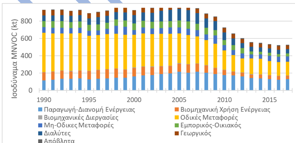
Γράφημα 25: Διαχρονική μεταβολή των εκπομπών προπομπών όζοντος στην Ελλάδα
