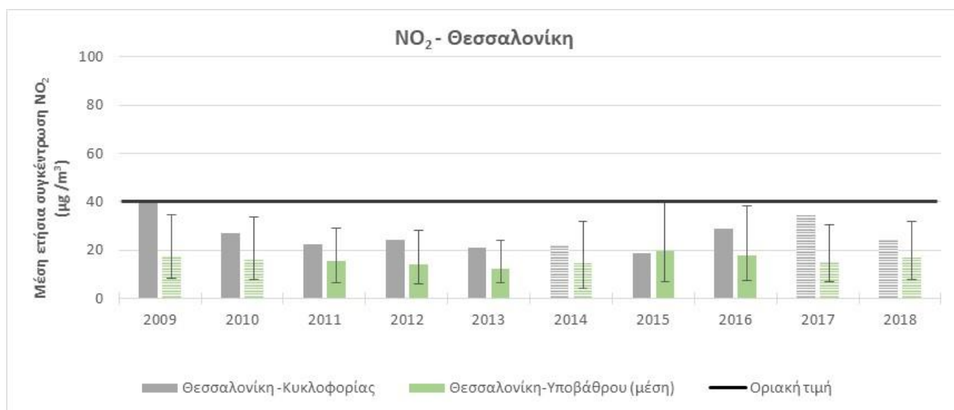
Γράφημα 44: Σύγκριση μέσης ετήσιας συγκέντρωσης NO 2 των σταθμών υποβάθρου και κυκλοφορίας στην ευρύτερη περιοχή Θεσσαλονίκης (2009-2018)
