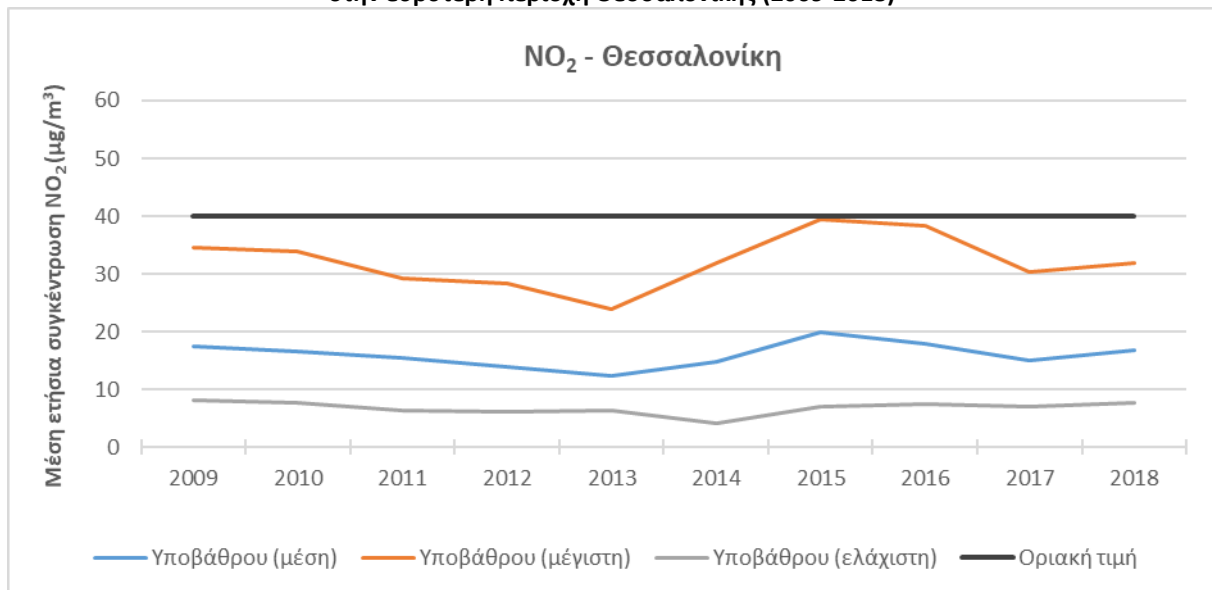
Γράφημα 41: Μέση ετήσια συγκέντρωση NO 2 των σταθμών υποβάθρου στην ευρύτερη περιοχή Θεσσαλονίκης (2009-2018)
