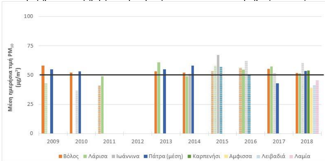
Γράφημα 47: Μέση ημερήσια συγκέντρωση PM 10 λοιπών αστικών περιοχών (2009-2018)
