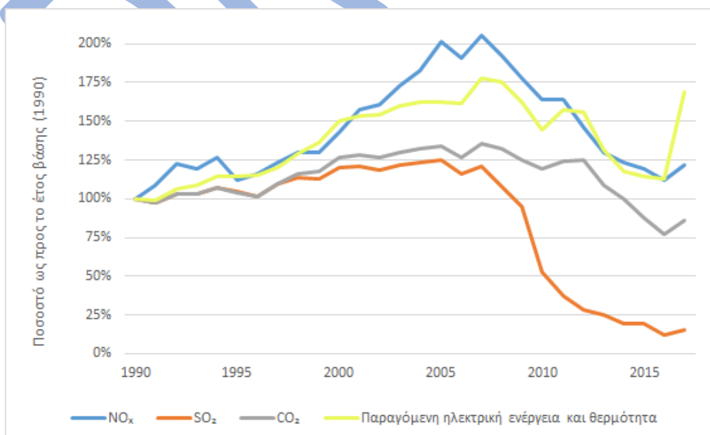
Γράφημα 35: Διαχρονική μεταβολή παραγωγής δημόσιας ηλεκτρικής ενέργειας και θερμότητας από ορυκτά καύσιμα και αντίστοιχες εκπομπές αέριων ρύπων
