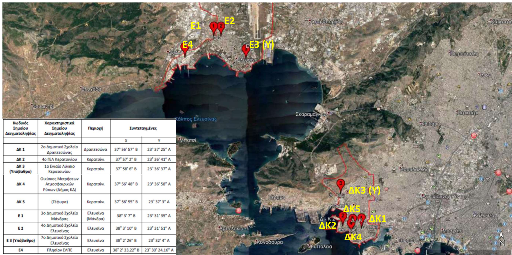
Εικόνα 2.1: Χωρική απεικόνιση των σημείων δειγματοληψίας VOCs στις περιοχές Δραπετσώνα-Κερατσίνι και Ελευσίνα.
